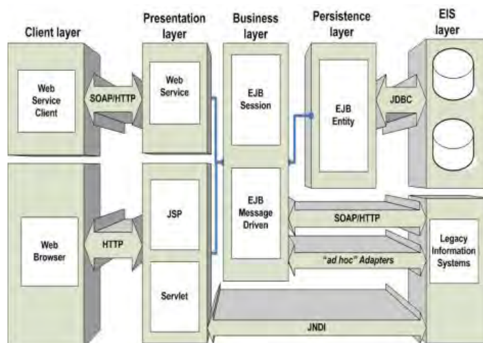
Figura52: Architettura del sistema informatico
